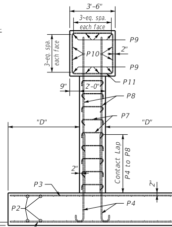
END ELEVATION
